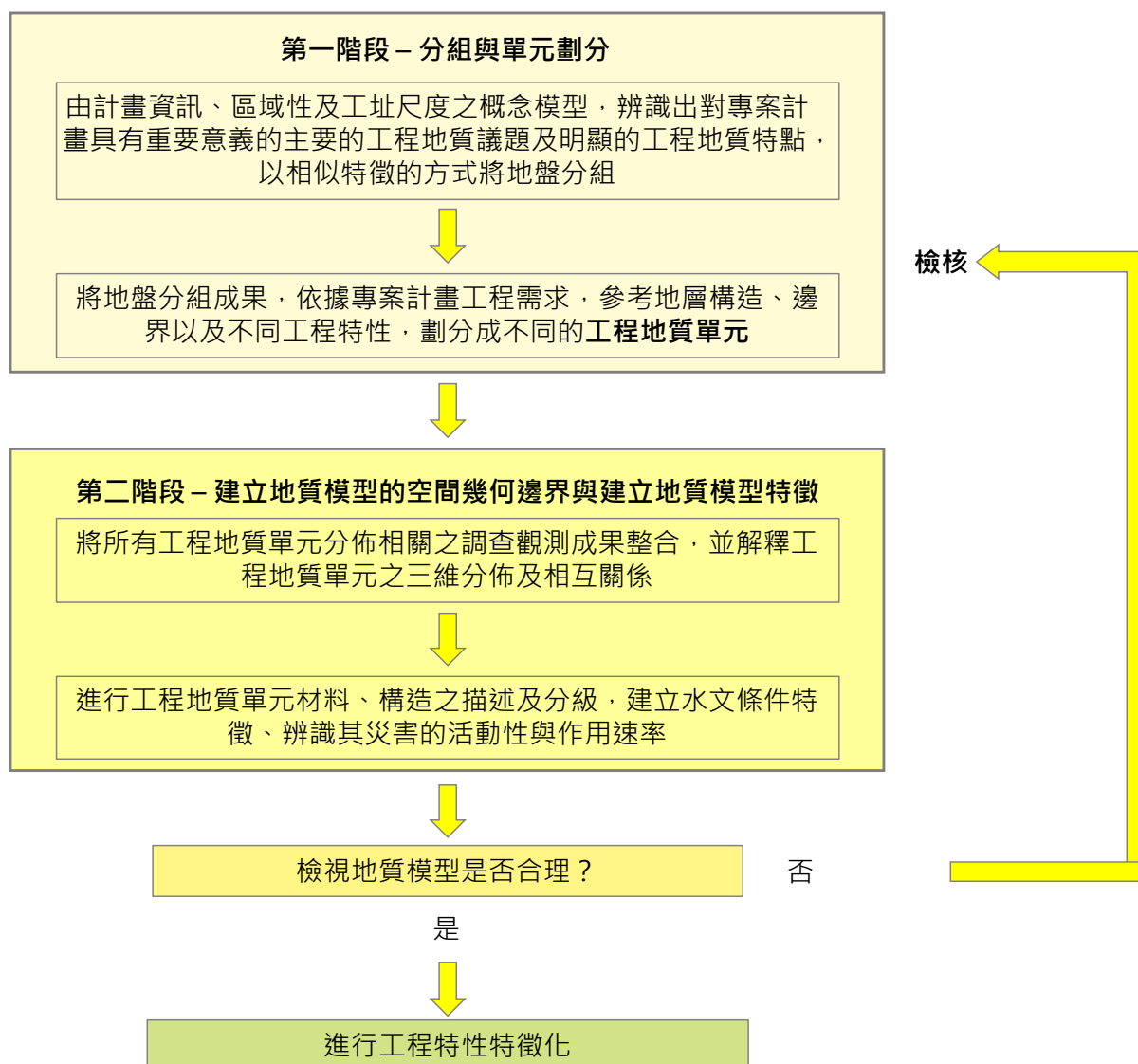
圖 1-4 建立工程地質單元及其作為地質模型之基礎
